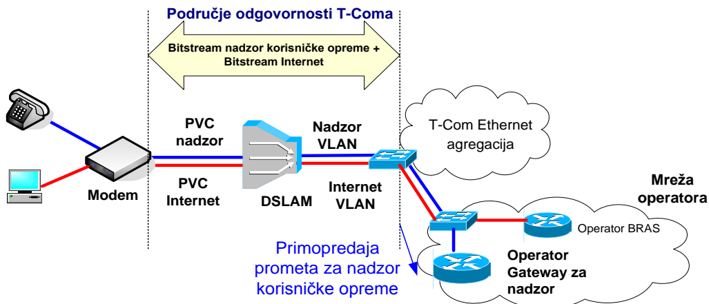
Slika 29. Veleprodajni širokopoljasi pristup za pružanje usluge nadzora korisničke opreme preko ADSL/VDSL pristupa na DSLAM razini
