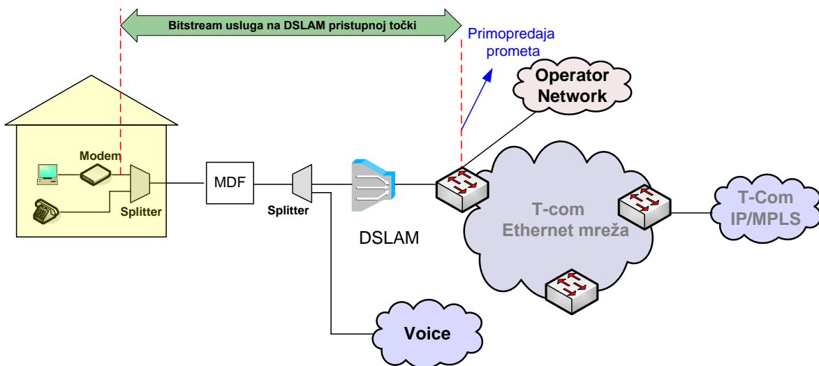
Slika 7. Veleprodajni širokopoljasn pristup za pružanje Internet usluge na DSLAM razini u slučaju kada krajnji korisnik ostvaruje Osnovni pristup mreži putem usluge HT-a
